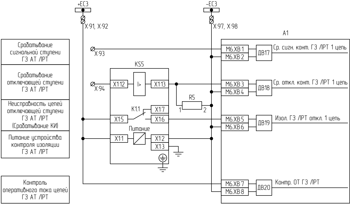
Цепи оперативного тока ГЗ АТ /РТ А1
